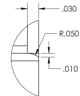
DETAIL D SCALE 8:1 12X TYP
